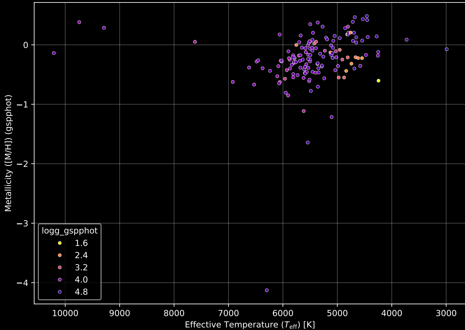
APOGEE DR17 Field: [044+54_MGA] Stellar Population Parameters (n= 148)
